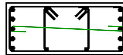
D 30 \times 70 10\varnothing 20 + 4\varnothing 14
