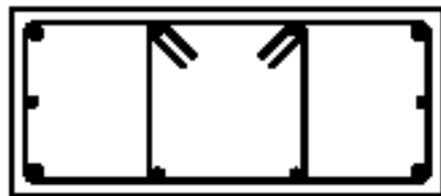
A 30 \times 70 4\varnothing 20 + 6\varnothing 14
